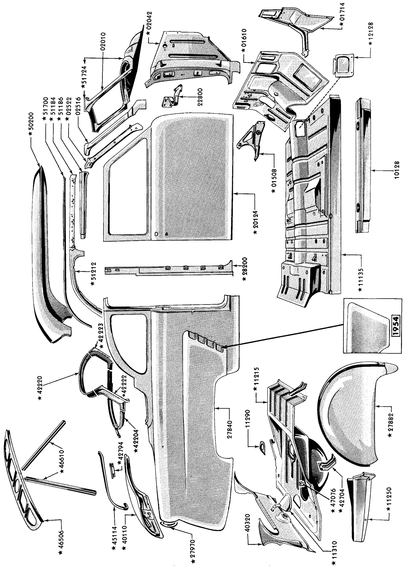
1953/54 COUPE (BODY TYPE 72)
