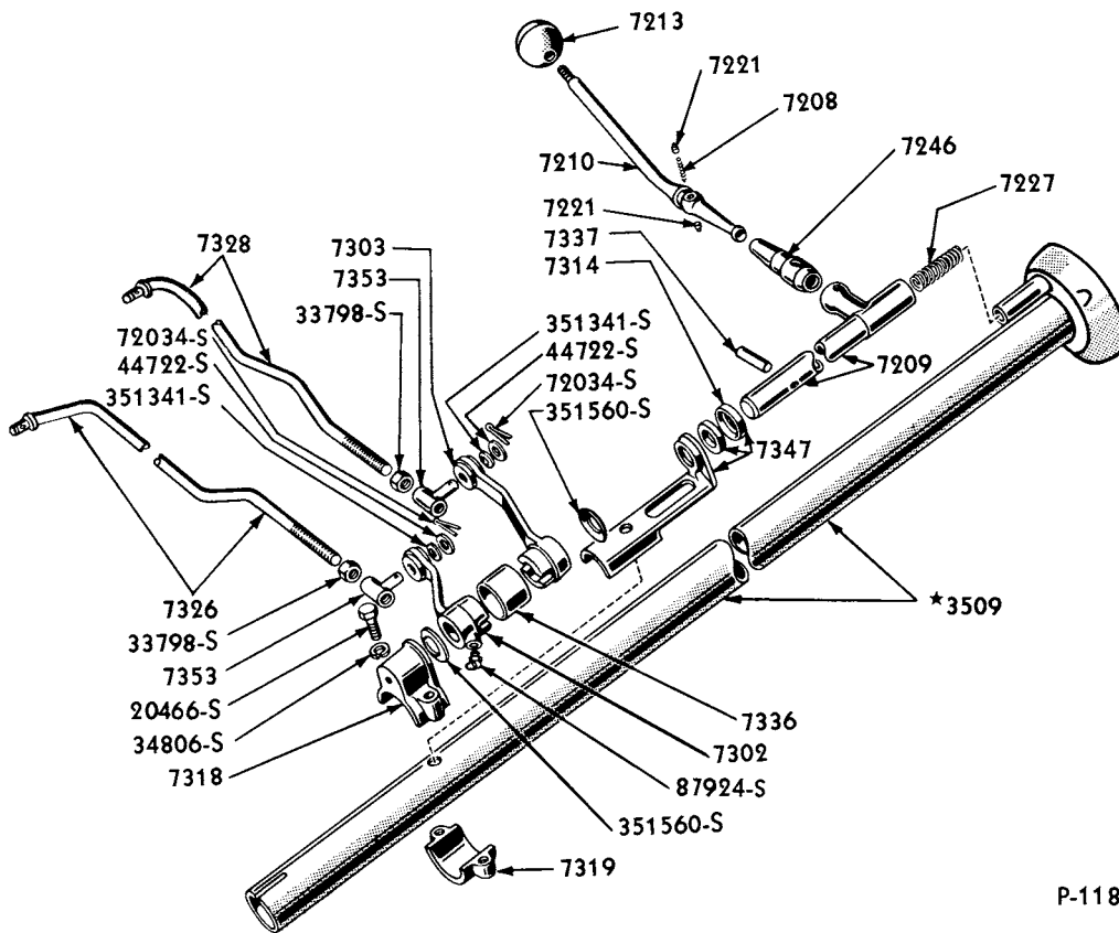
1951 GEAR SHIFT COLUMN
