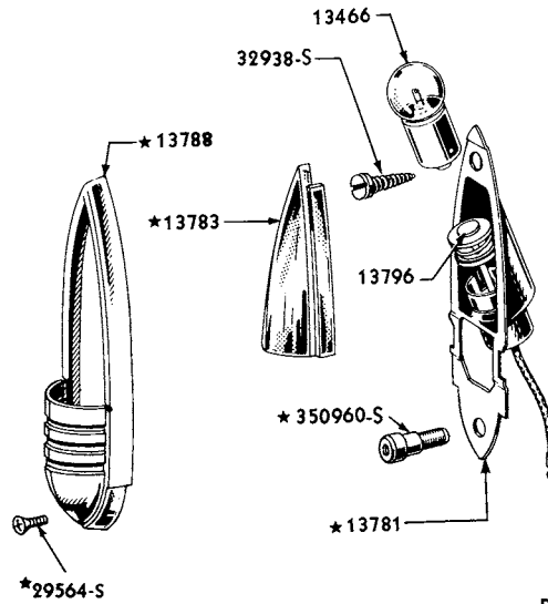
1950 TUDOR SEDAN PILLAR LAMP
