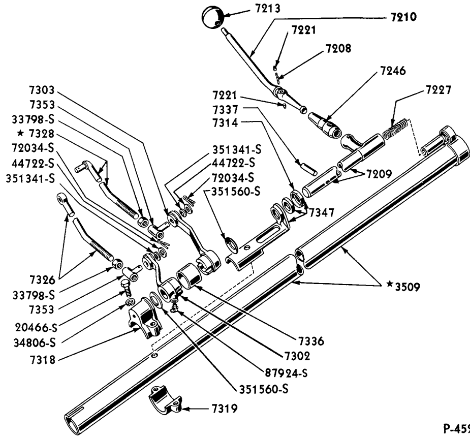
1949/50 GEAR SHIFT COLUMN
