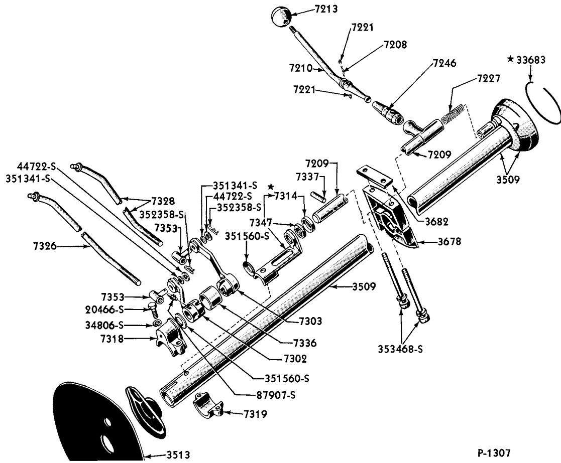
1952/53 GEAR SHIFT COLUMN
