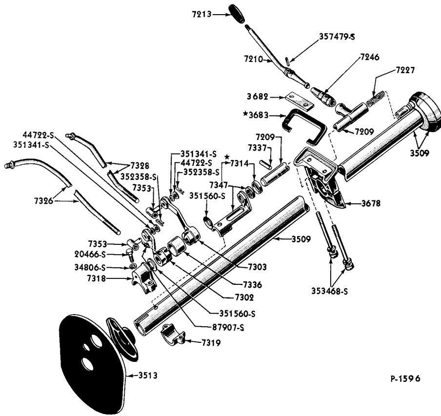
1954 GEAR SHIFT COLUMN
