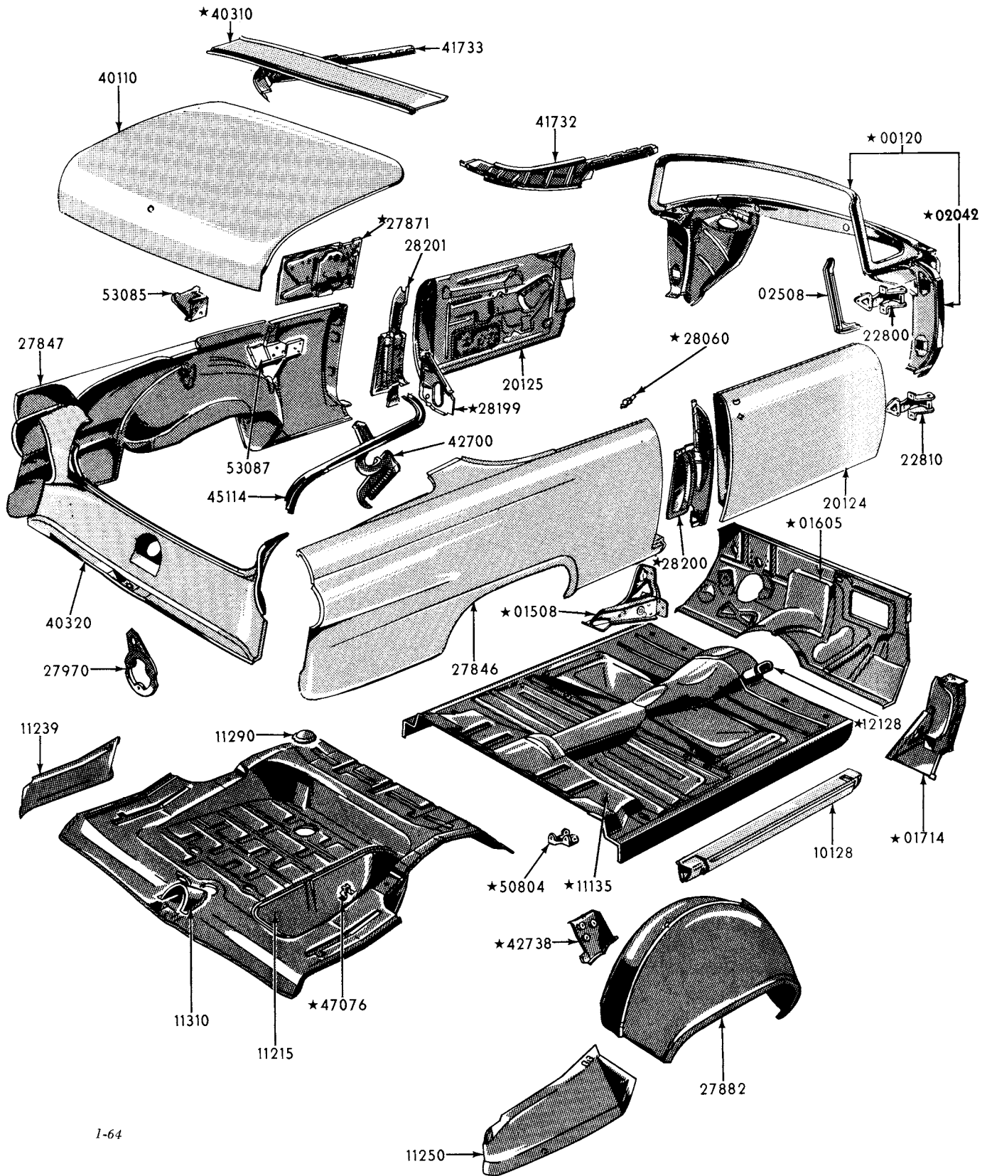
1955/56 FAIRLANE CONVERTIBLE COUPE (BODY TYPE 76B)
